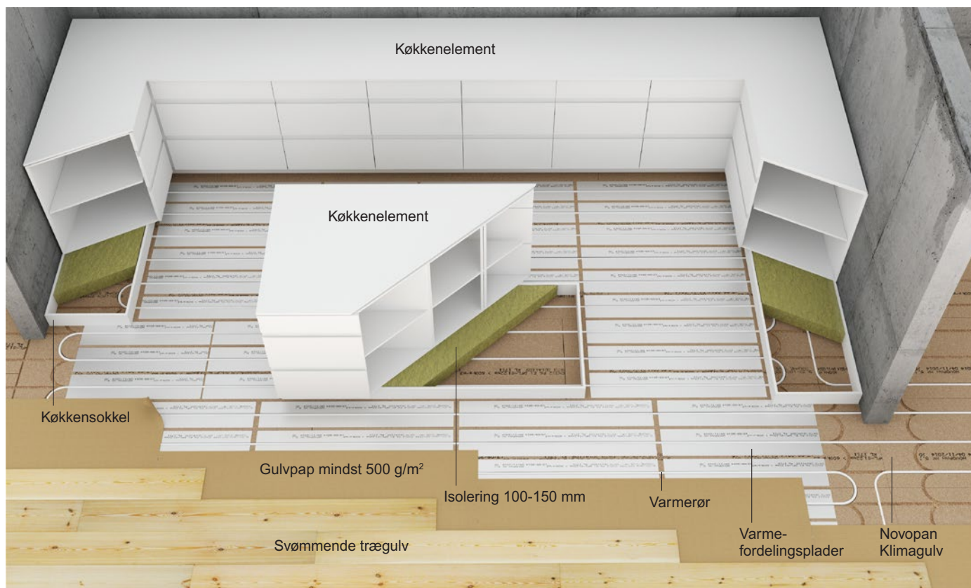
Figur 1 Placeringen af køkkenskabe tegnes på betondækket, så vendespor kan udføres under soklerne.
