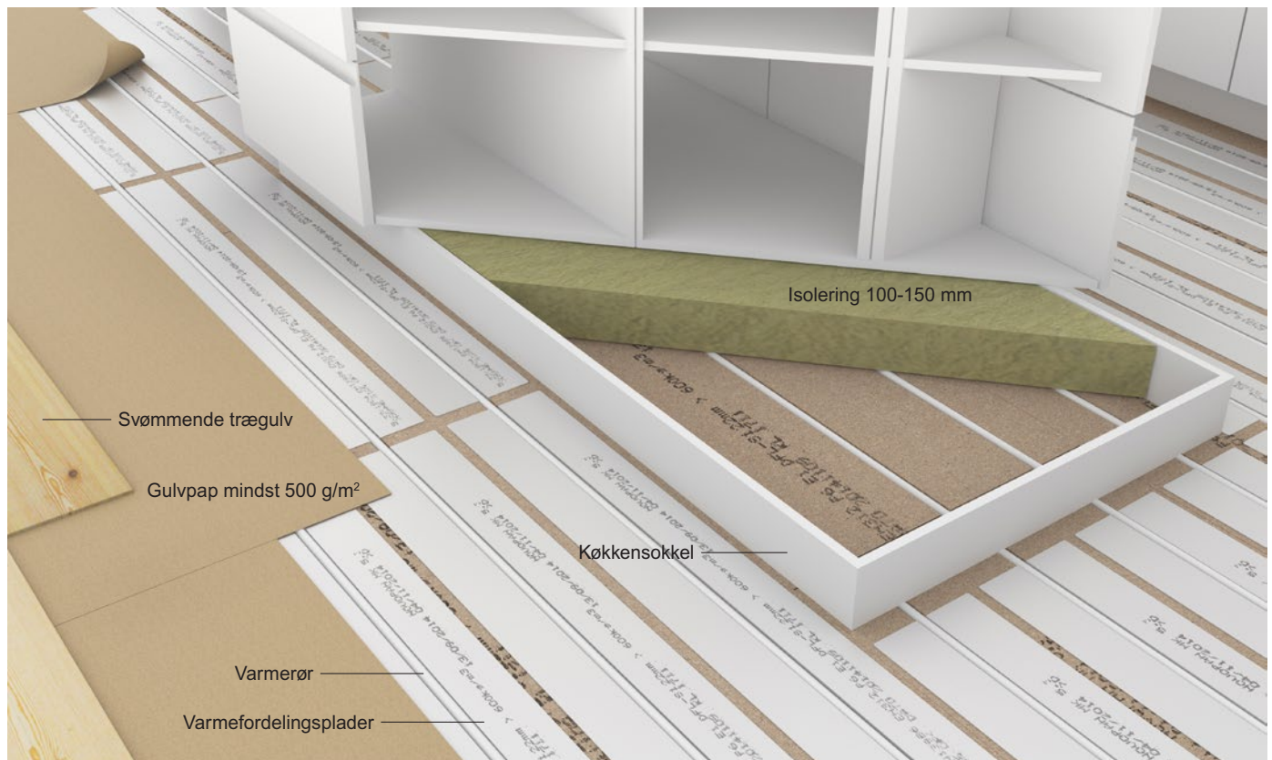
Figur 2 Sokler under køkkenskabe skal isoleres med 100-150 mm mineraluld for at undgå opvarmning af sokkelrummet.
